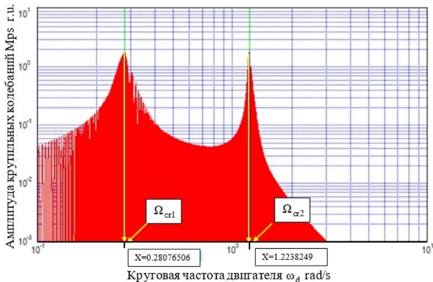
Рисунок 4 ЛАЧХ трехмассовой части пропульсивной установки
