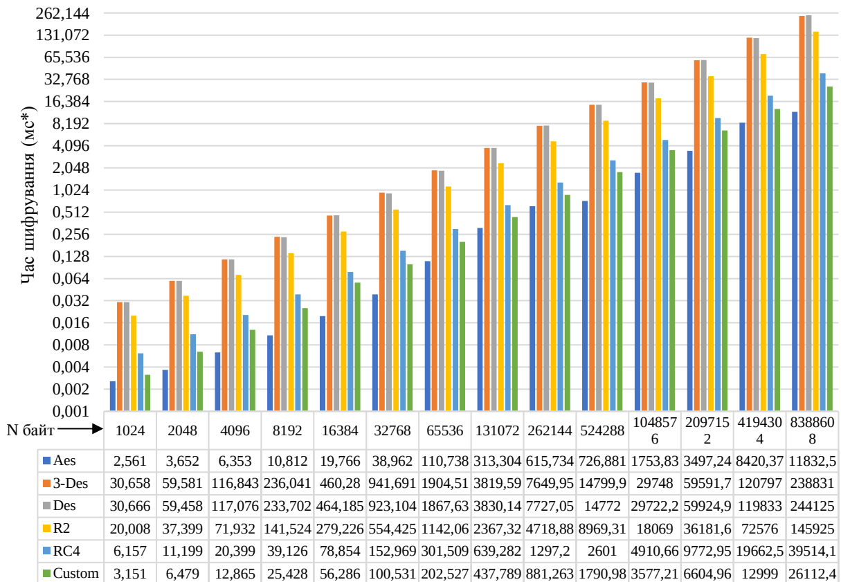
Рис. 1 Швидкість шифрування (мс) N байт
