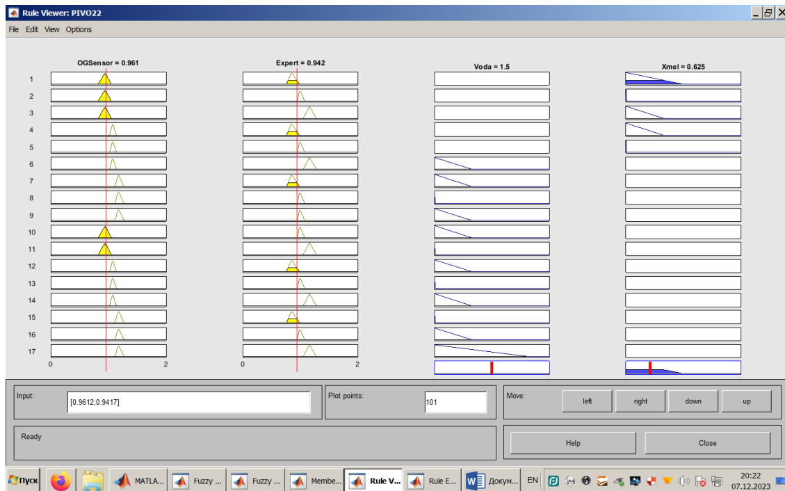
Рис. 2. Вікно Rule Viewer для використання оператором при прийнятті рішення щодо керування щільністю пива
