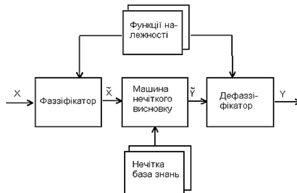
Рис. 1. Типова архітектура системи нечіткого висновку
